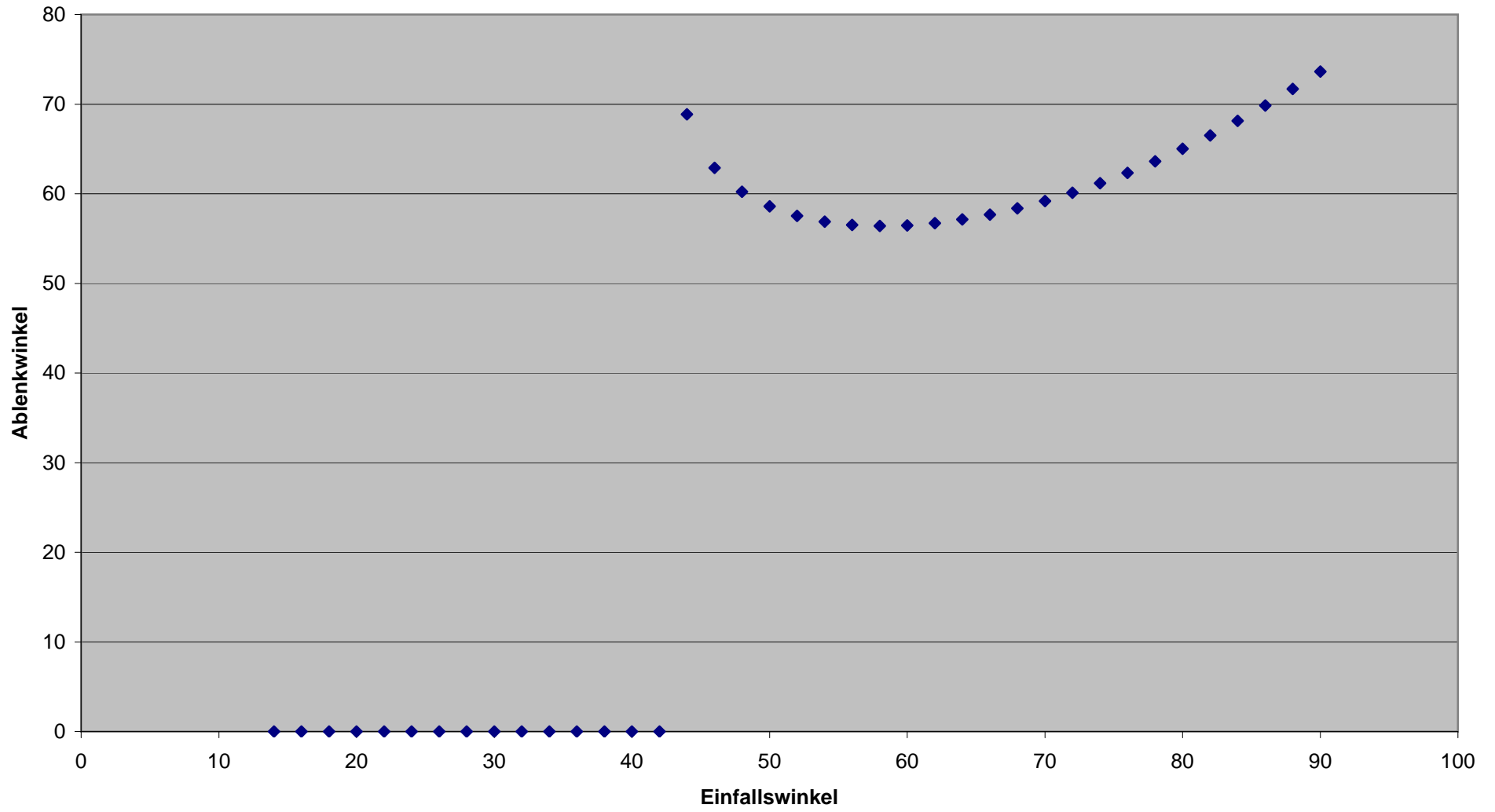
Gesamtablenkung bei \epsilon=60^\circ
