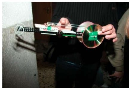
165 Mausefallenautowettbewerb; Privat
